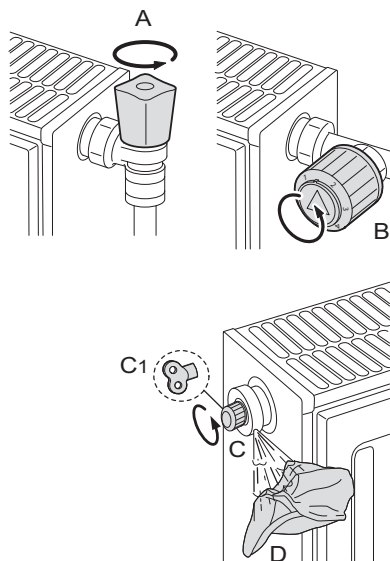
Fig.10 Purga de la instalación
