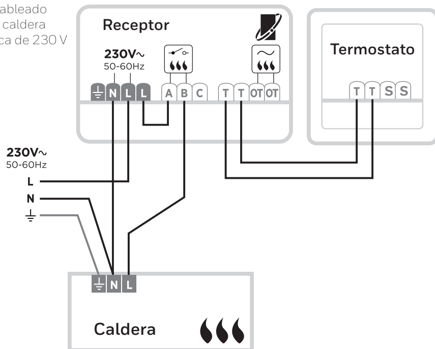
B) Cableado para caldera combi
